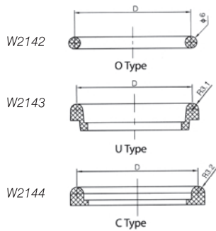
○型密封圈 O-ring
