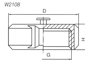
长型圆螺母 / 盲螺母 (可带链条) Long round nut / Blind nut (available with chain)
