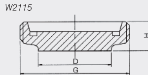
DIN 盲螺纹接头 DIN Blind male
