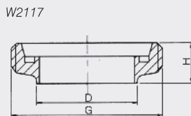
DIN11850 系列 0&2 短螺纹接头 DIN11850 series 0&2 Short male
