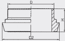
DIN11851 长厚型平接头 DIN11851 Long liner
