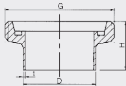
DIN11850 系列 O&2 长型螺纹接头 DIN11850 Series O&2 Long male
