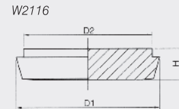
DIN 盲平接头 DIN Blind ferrule
