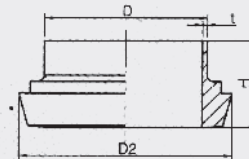
DIN11850 系列 O&2 长型平接头 DIN11850 Series O&2 Long liner
