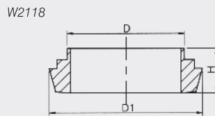
DIN11850 系列 0&2 短型台阶型平接头 DIN11850 series 0&2 Short Stepped liner
