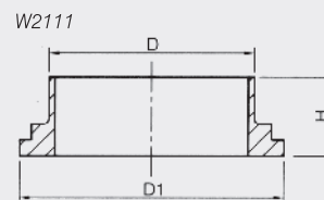
长型平接头 (台阶型) Long stepped liner
