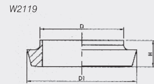
DIN11850 系列 0&2 短型平接头 DIN11850 series 0&2 Short Liner
