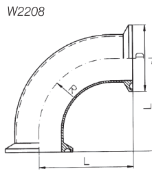
W2208 DIN 卡箍式弯头 (90° ) DIN Clamp Elbow (90° )
