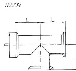
W2209 DIN 卡箍式三通 DIN Clamp Tee
