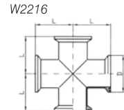
INCH 卡箍三通 / 卡箍四通 INCH Clamp Tee/Clamp Cross
