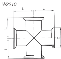
W2210 DIN 卡箍式四通 DIN Clamp Cross
