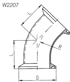
W2207 DIN 卡箍式弯头 (45° ) DIN Clamp Elbow (45° )
