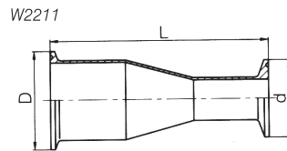
W2211 DIN 卡箍式同心大小头 DIN Clamp Concentric Reducer
