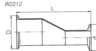
W2212 DIN 卡箍式偏心大小头 DIN Clamp Eccentric Reducer
